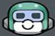
GitHub Copilot
